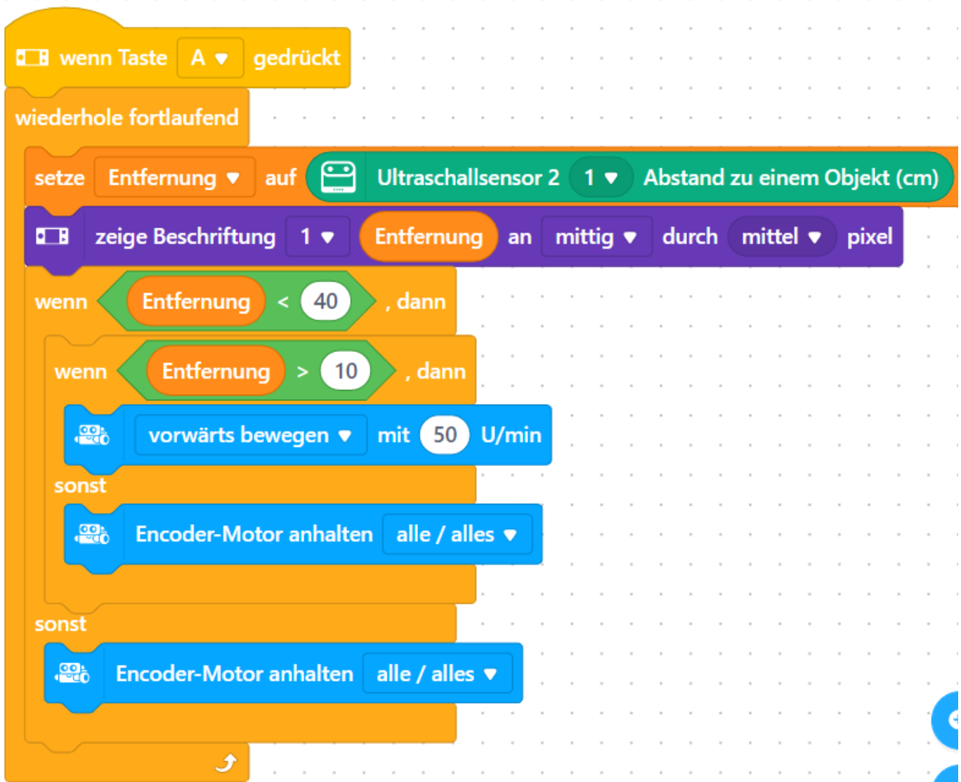
Abbildung 45: Roboter folgt einem Objekt
