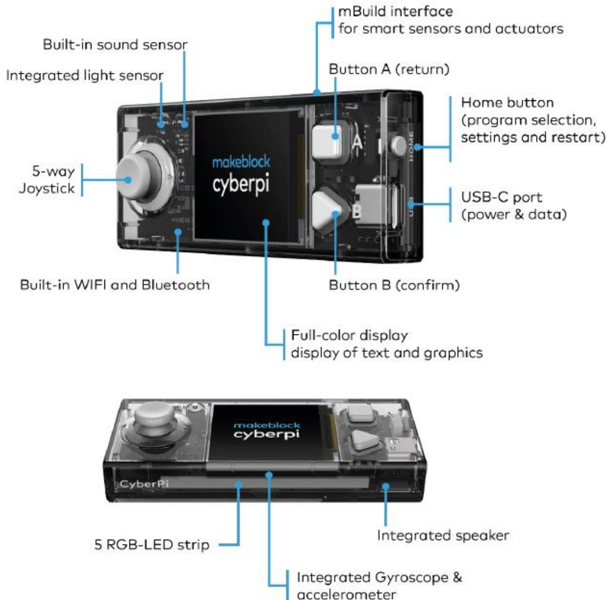
Abbildung 33: CyberPi – Funktionen
