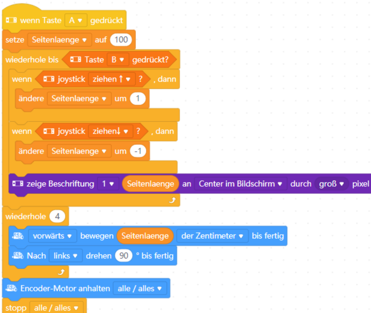
Abbildung 44: Lösung der Quadrataufgabe mit variabler Seitenlänge
