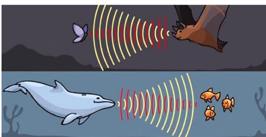
Abbildung 38: Ultraschall in der Tierwelt
