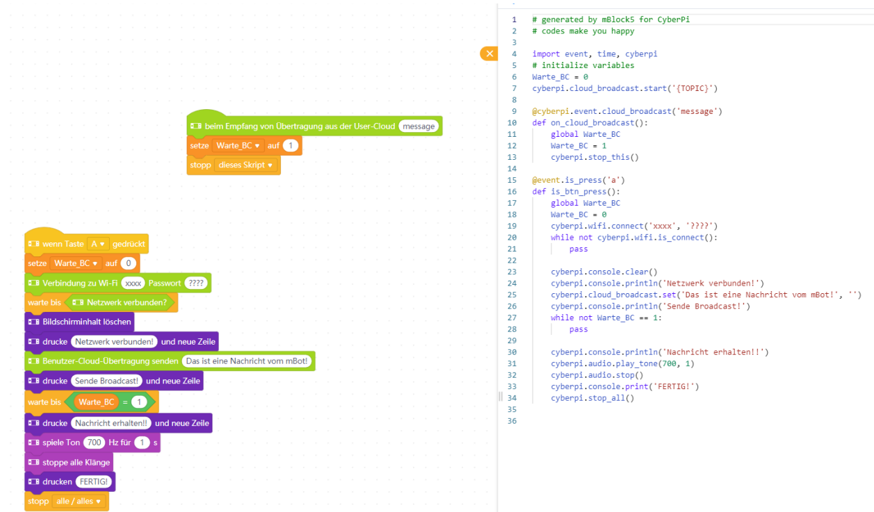
Abbildung 7: Block- oder Pythonoberfläche?
