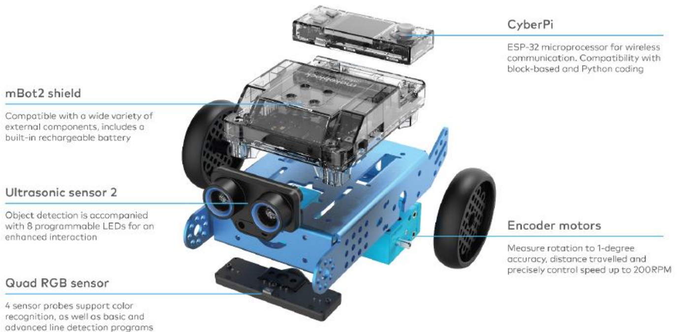
Abbildung 2: mBot2 - Grundstruktur
