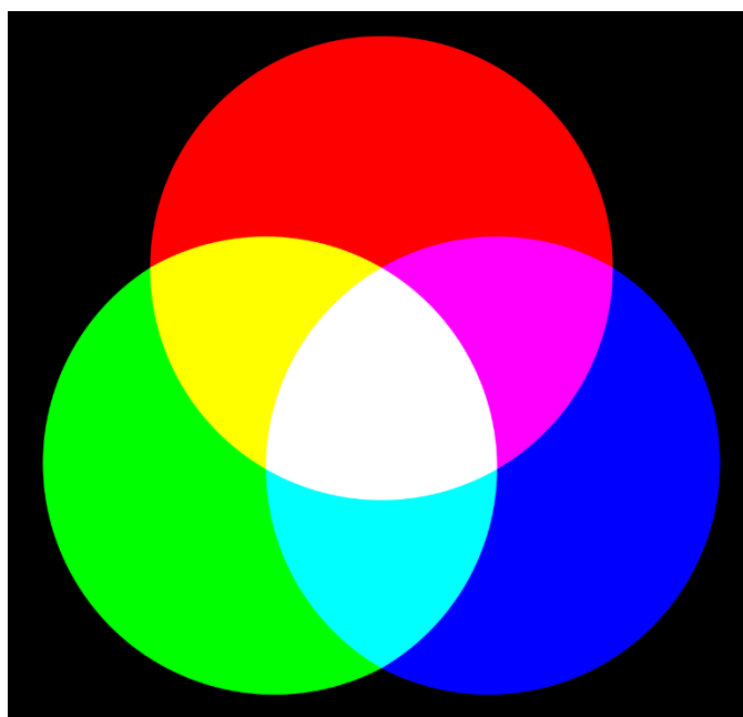
Abbildung 50: Prinzip der additiven Farbmischung
